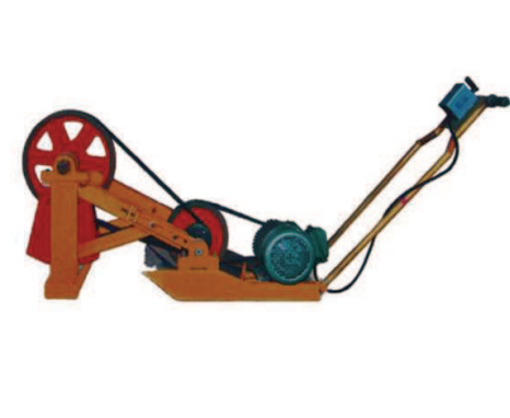
Fig. 4 the inertia rammer
