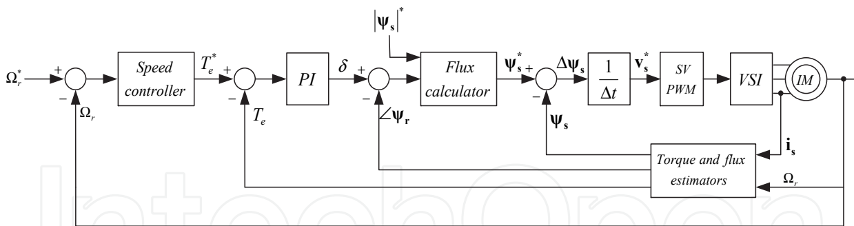
Fig. 9. DTC-SVM scheme
