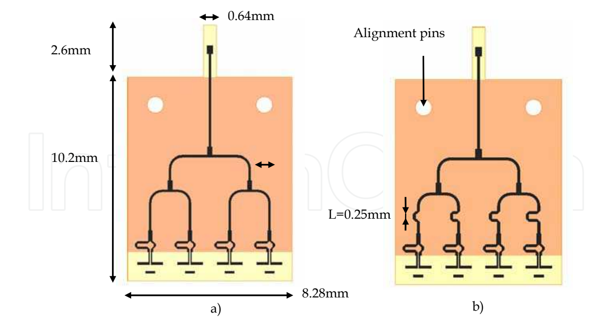
Fig. 14. Layouts of: a) Array-0°, and b) Array-57°
