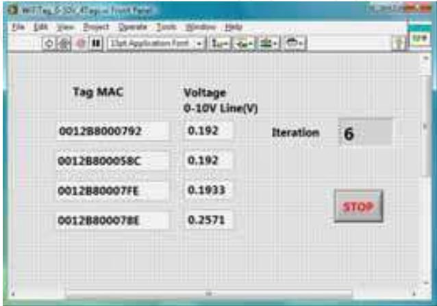
Fig. 11. WiFiTag_0-10V_4Tags VI
