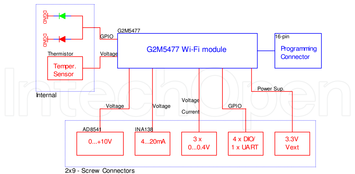
Fig. 2. Tag4M Bloc Diagram
