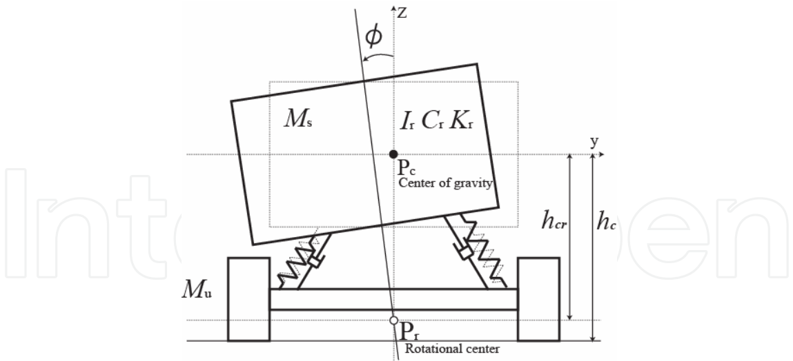
Fig. 4. Rolling model
