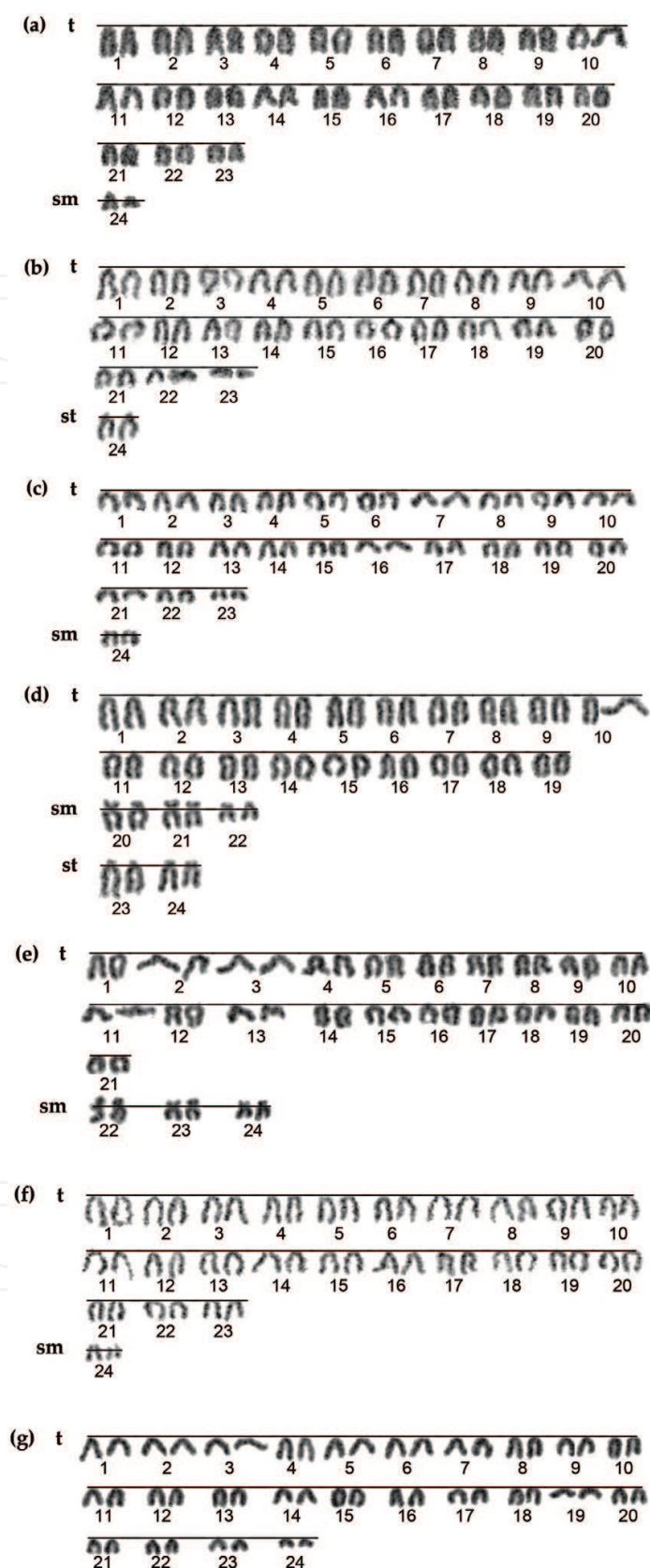
Figure 2. Karyotype analyses of seven groups: (a) Epinephelus coioides ; (b) E. flavocaeruleus ; (c) E. fuscoguttatus ; (d) E. lanceolatus ; (e) E. polyphkadion ; (f) E. tukula ; and (g) Plectropomus leopardus .
