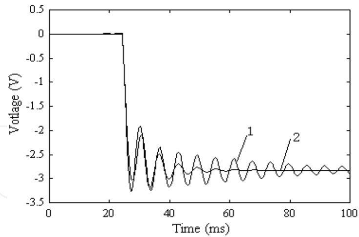
(d) Channel M_x
