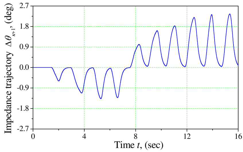
Fig. 21. Impedance trajectory
