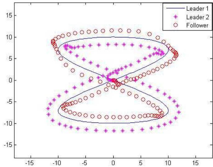
Fig. 13. Actual trajectory using separation-separation controller for Eq. (46)
