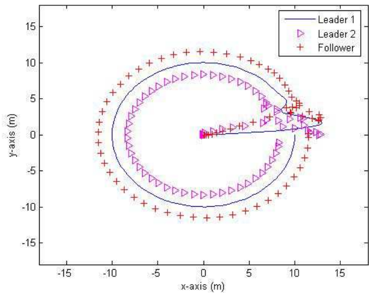
Fig. 12. Actual trajectory using separation-separation controller for Eq. (44)
