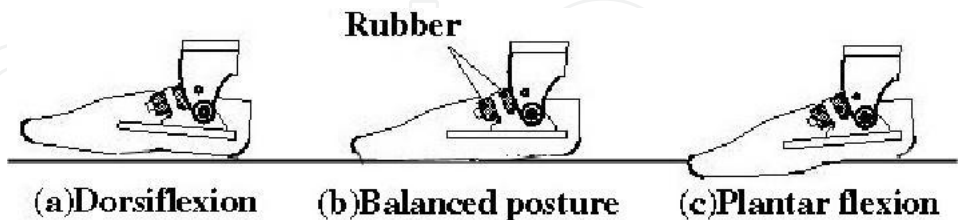
Fig. 29. Prosthetic foot.
