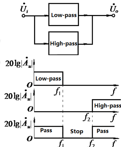
(d) Band elimination filter principle diagram
