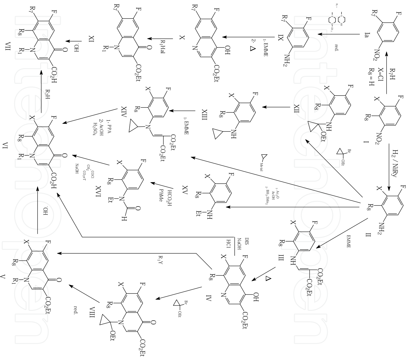
Fig. 11. Gould-Jacobs method.
