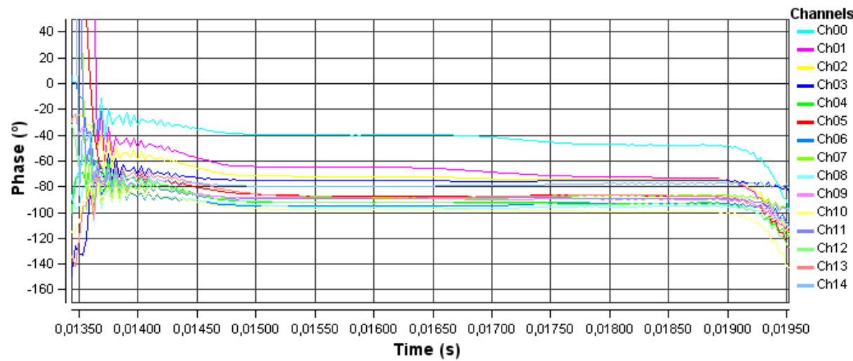
Fig. 4.2. Rx phase values
