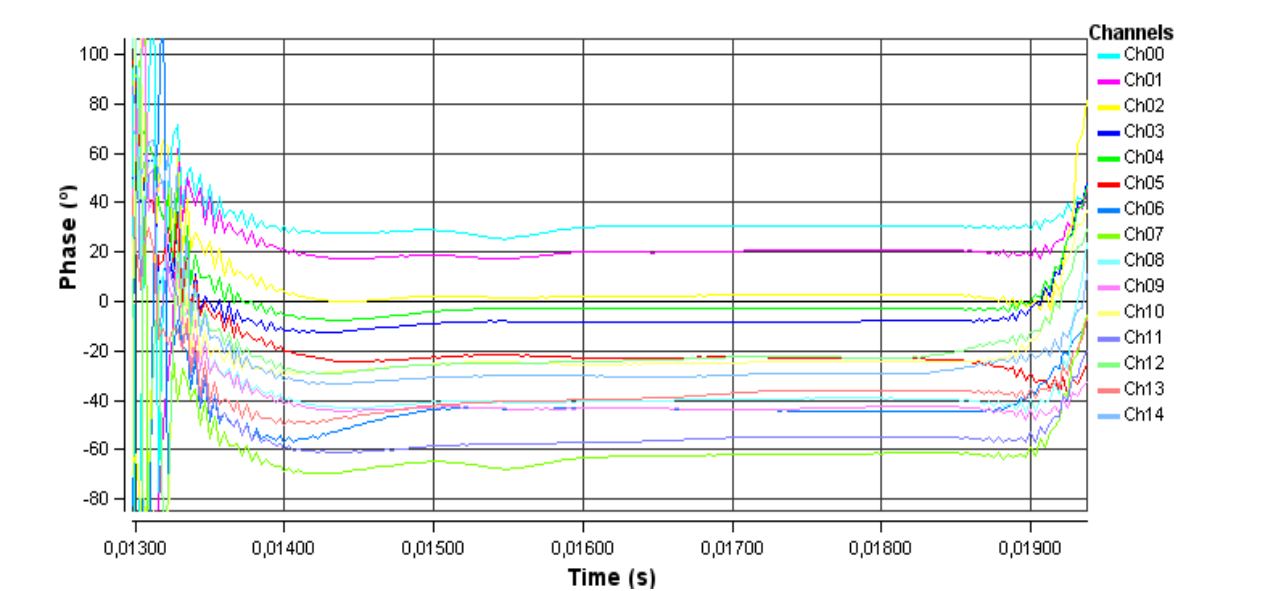
Fig. 3.3. Tx phase values
