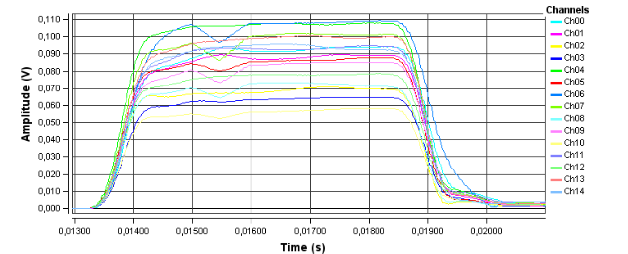
Fig. 3.2. Tx module values
