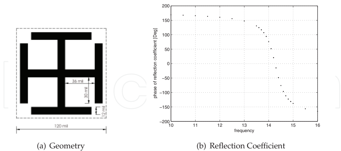
Fig. 10. UC-EBG
