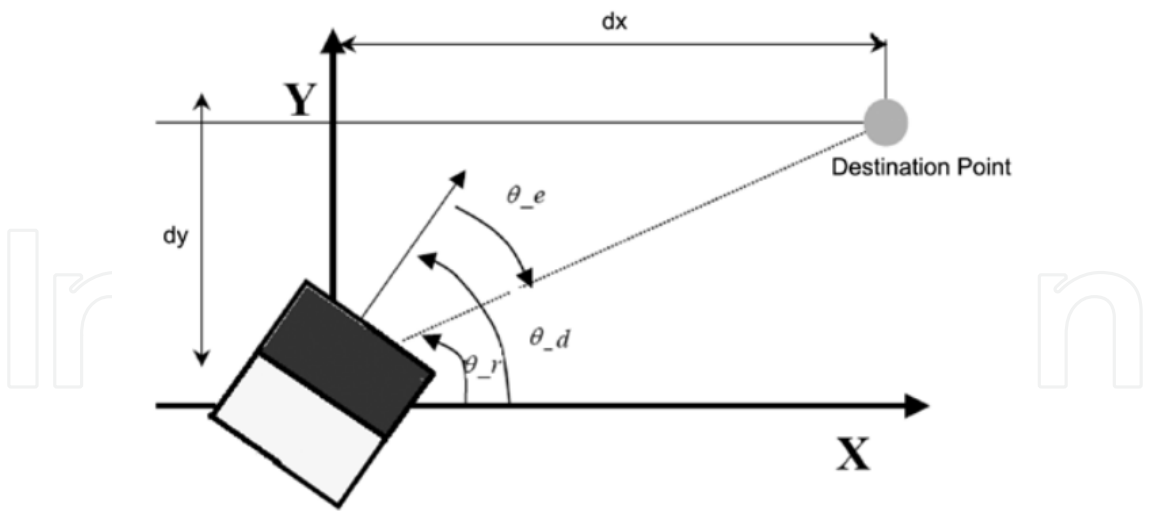
Fig. 24. Parameter defined for mobile robot
