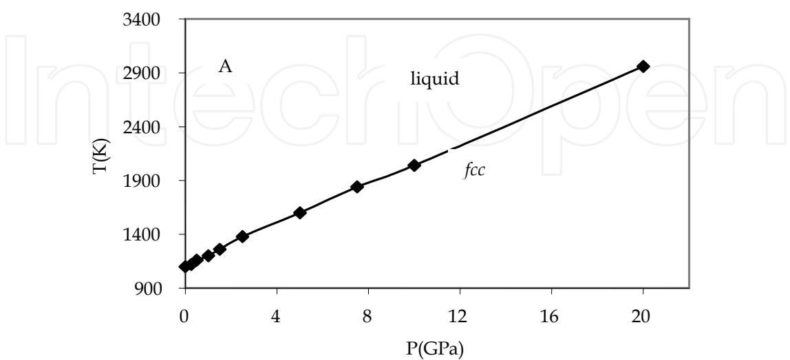
Fig. 6. P-T diagrams for Au.
