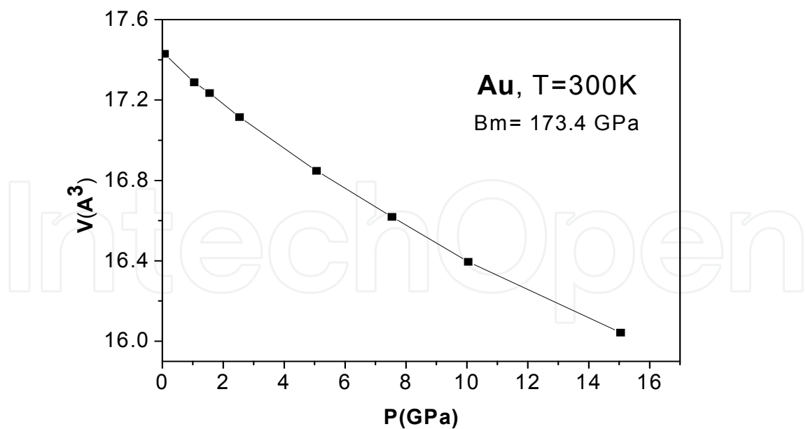
Fig. 2. P-V diagrams for Au.
