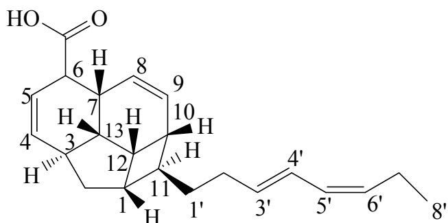
35: Erythrophloin E
