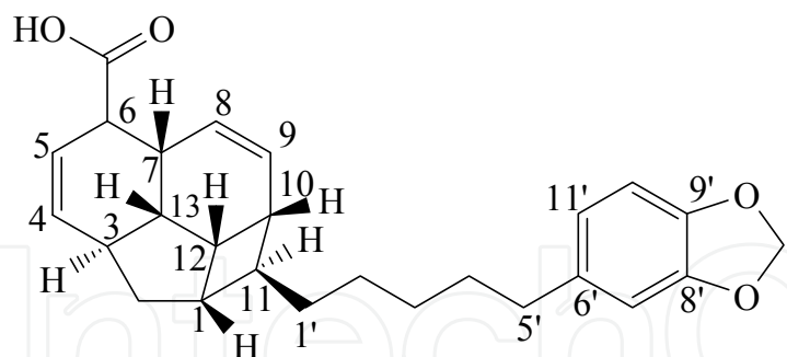
33: Erythrophloin F
