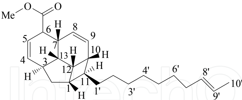
37: Erytrophloin D
