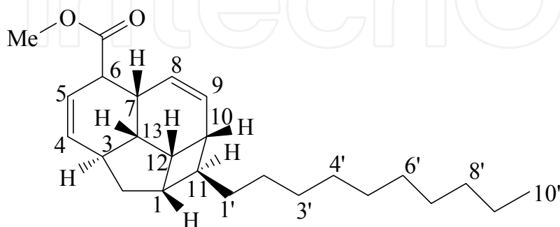
36: Erythrophloin B
