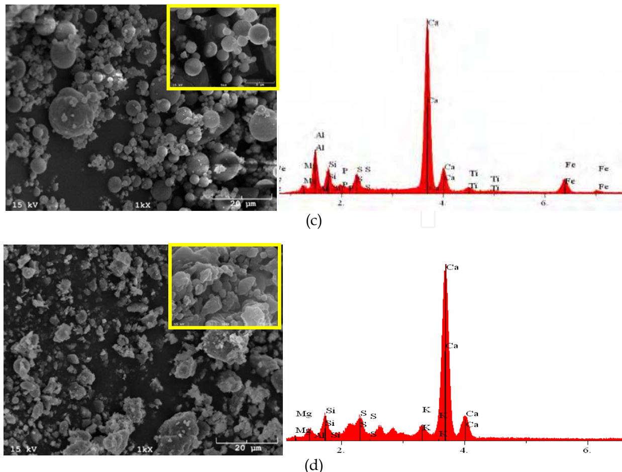
Fig. 4. SEM/EDS of (a) Raw Soil (b) Lime, (c) CFA, and (d) CKD Powder
