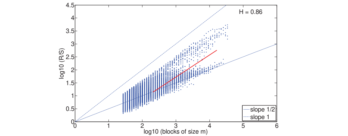
Fig. 4. Hurst Parameter Estimation via the R/S Method.
