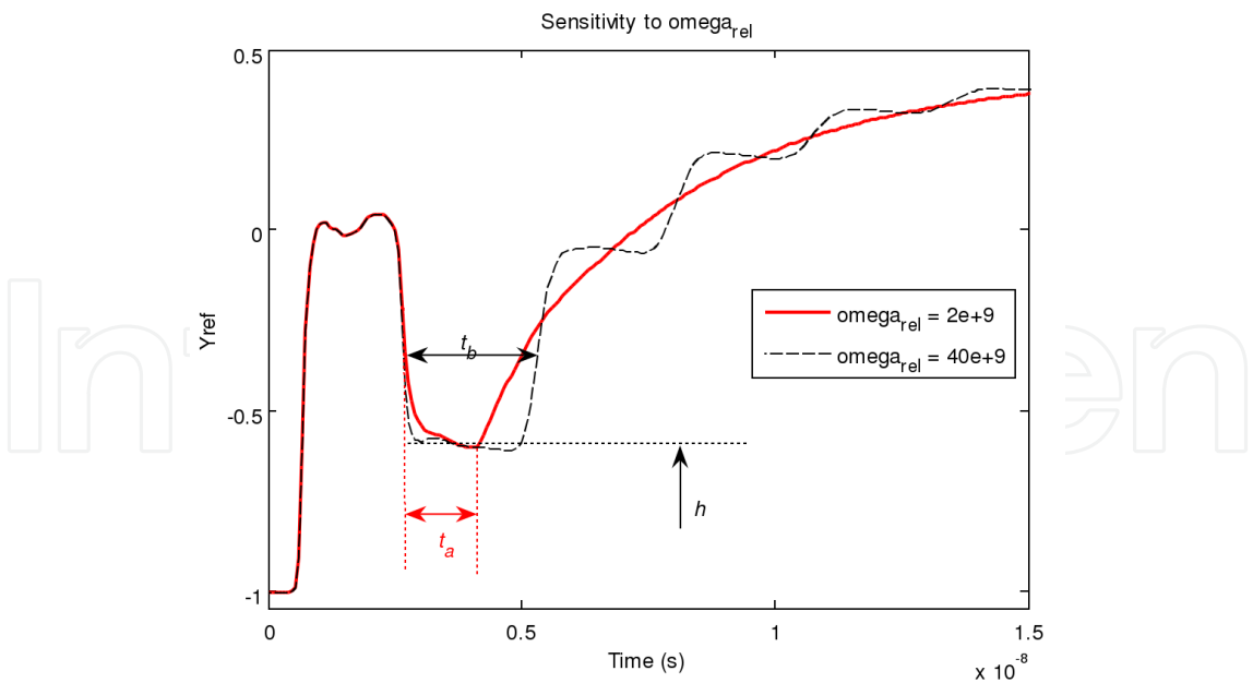
Fig. 14. Definition of the parameters h, t_a, t_b .
