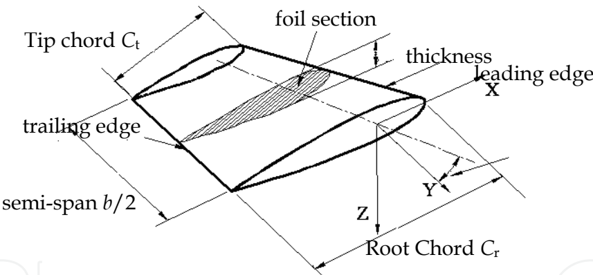
Fig. 13. Rudders parameters
