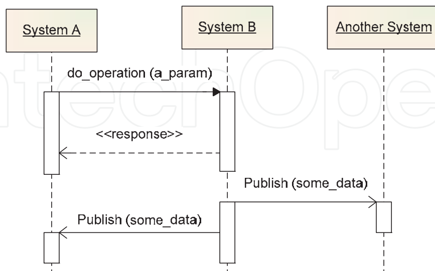
Fig. 11. Interaction Scenario.
