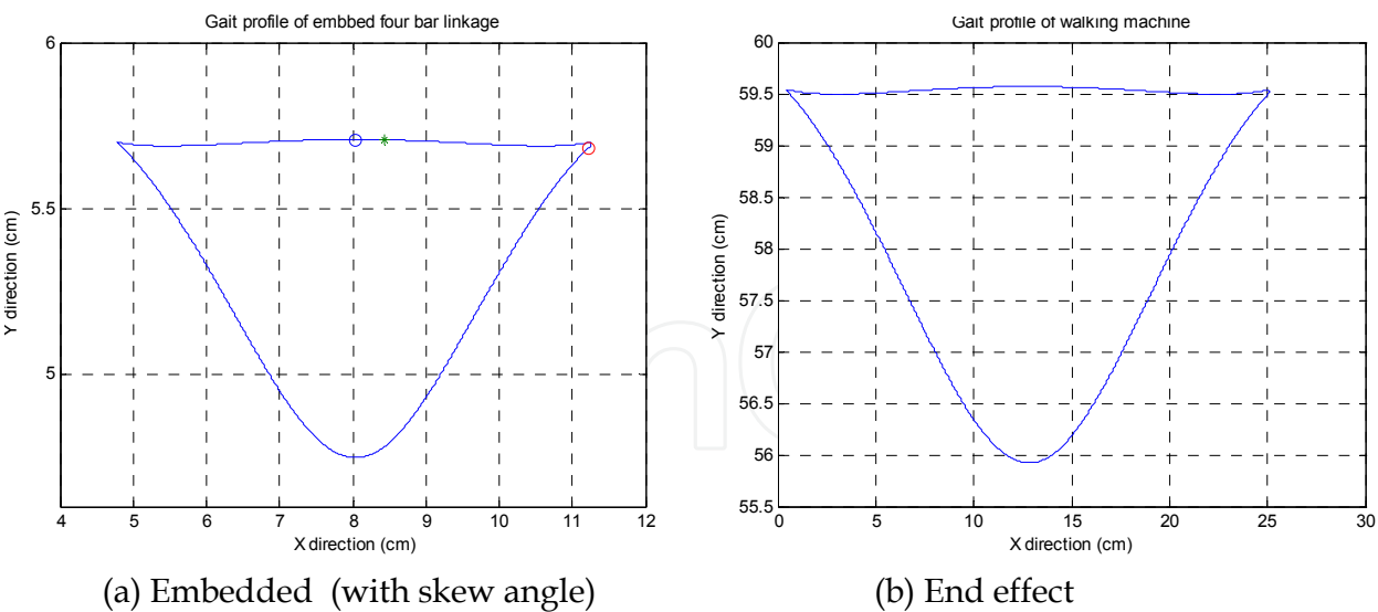
Fig. 6. Gait profile.
