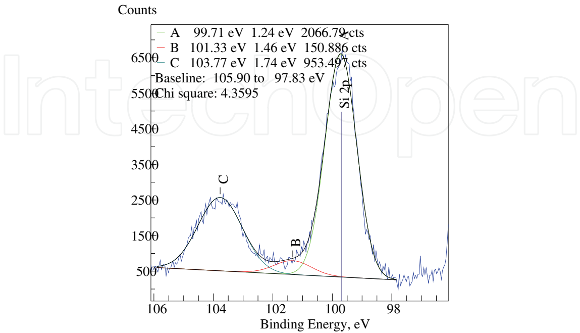
Fig. 3. Si 2p spectra for Si 4+ (SiO 2 -A) and Si 0 (bulk-C)
