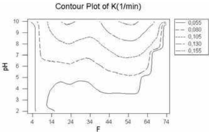
Fig. 12. Contour Surface, ABr 75, T i =45 °C, 15<TO<150
