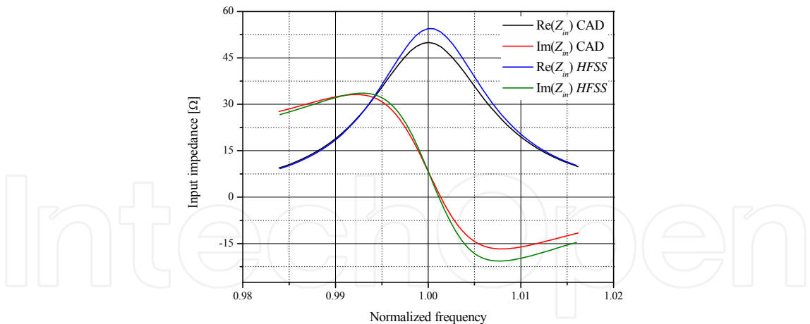
Fig. 24. Input impedance.
