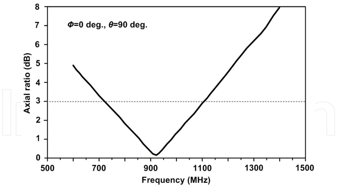
Fig. 12. AR spectrum
