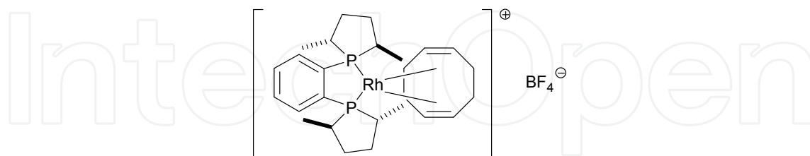
Fig. 27. Rh-MeDuPHOS ( 24 )
