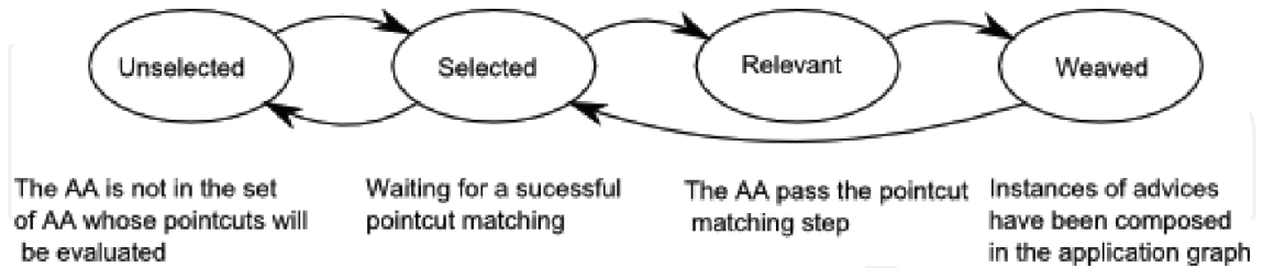
Fig. 18. AA life cycle
