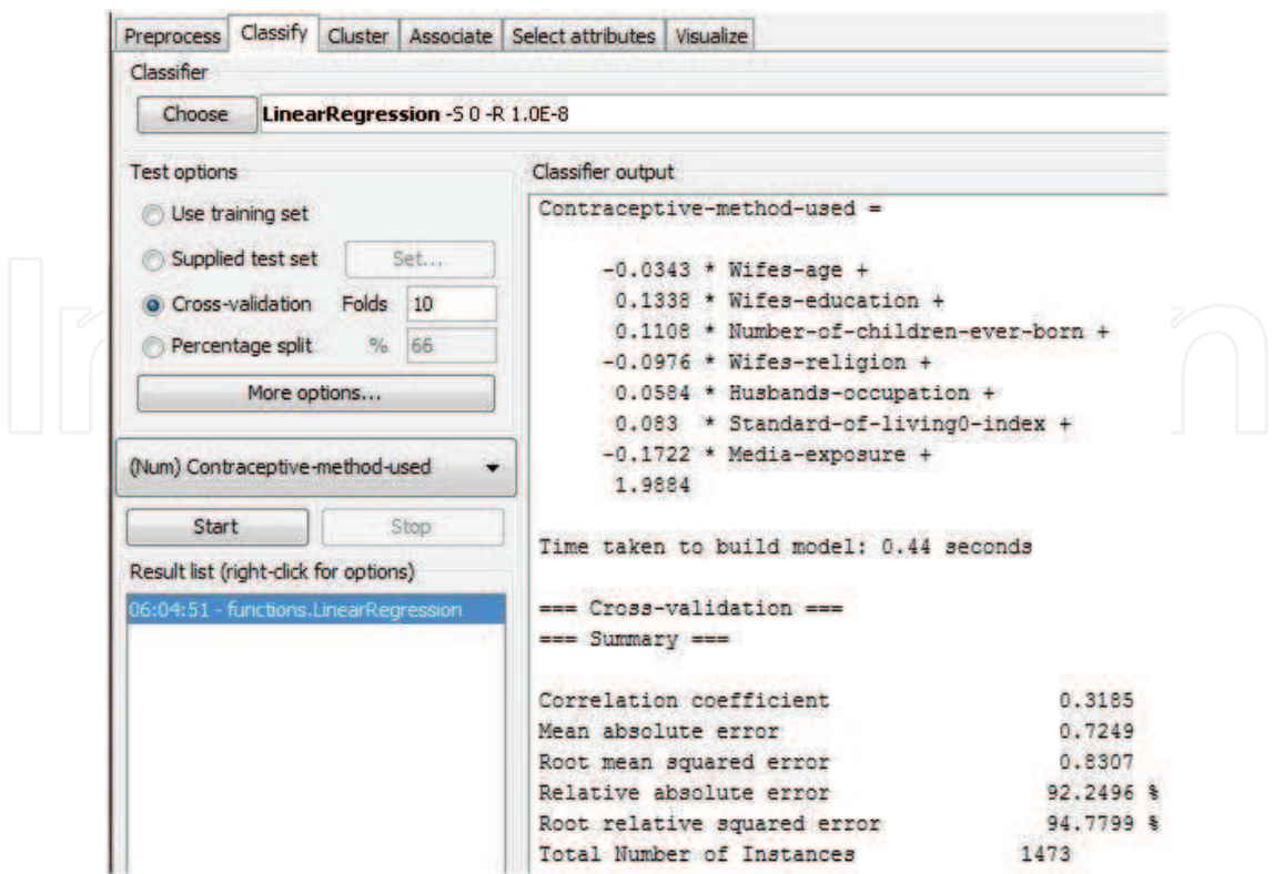
Fig. 13. Output of Weka.
