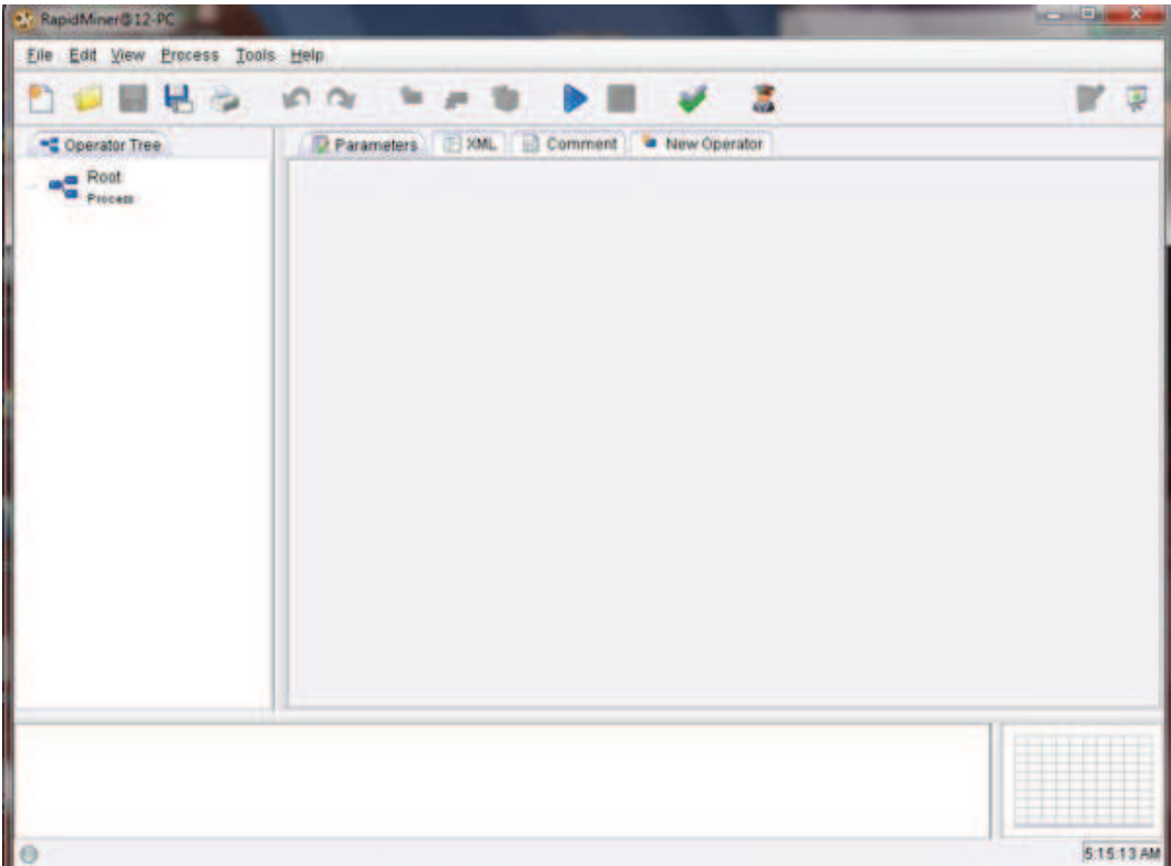
Fig. 14. Rapidminer enviroment.
