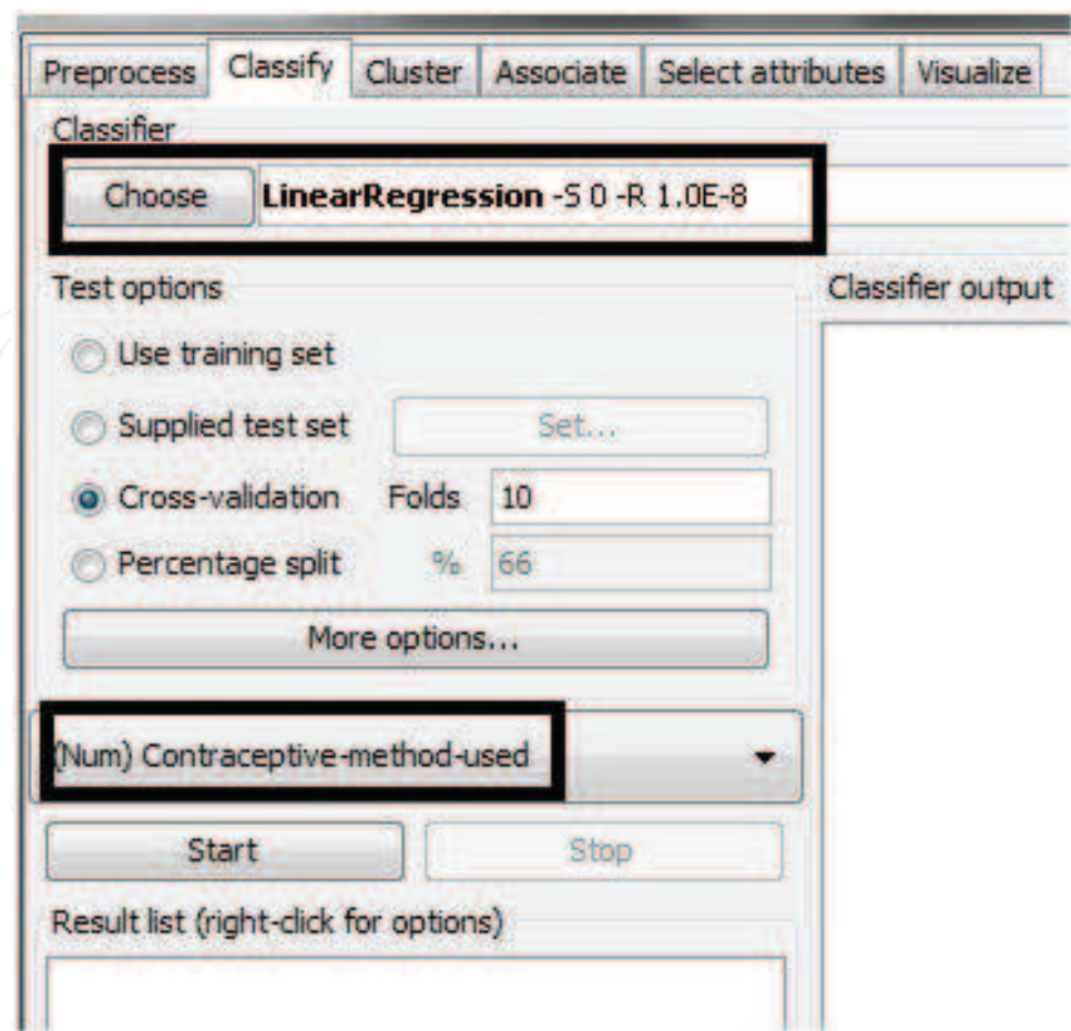
Fig. 12. Classify.
