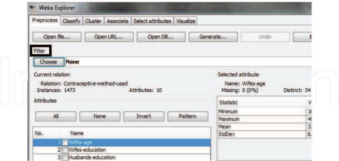
Fig. 11. Filter.
