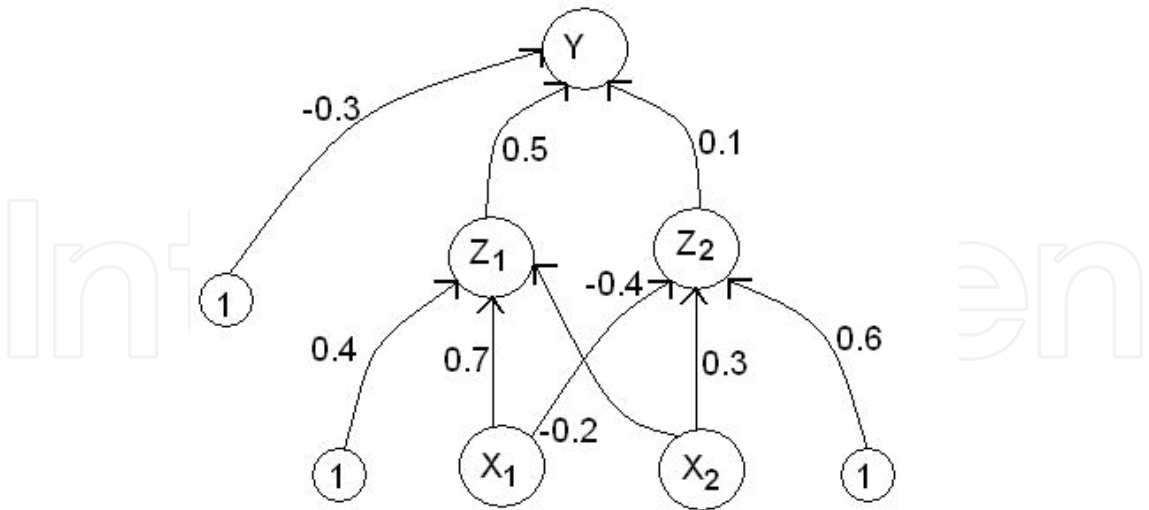
Fig. 9. MLP.
