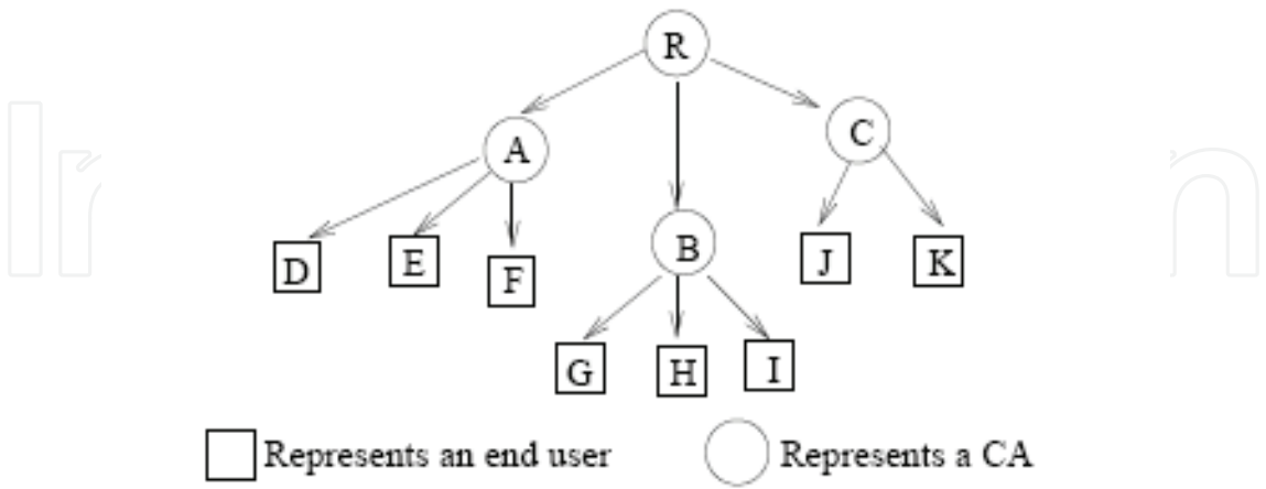
Fig. 3. Hierarchical trust
