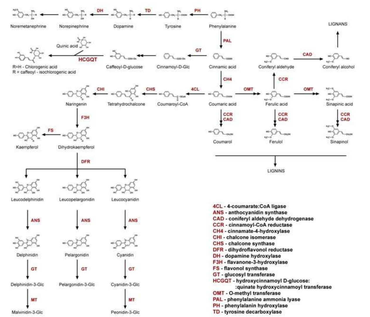
Fig. 7. The phenylpropanoid pathway
