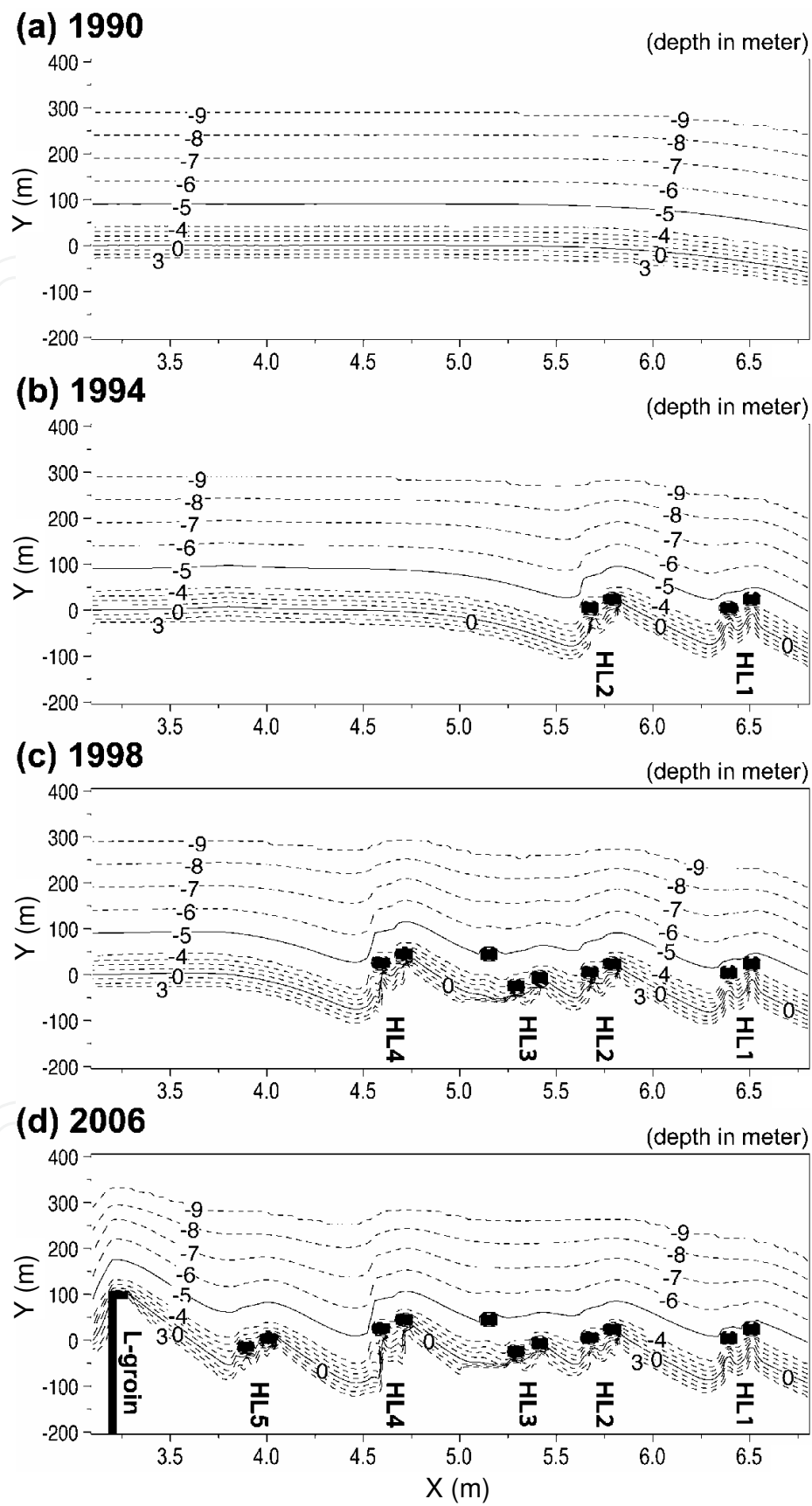
Fig. 25. Predicted bathymetries ((a) 1990, (b) 1994, (c) 1998, and (d) 2006)
