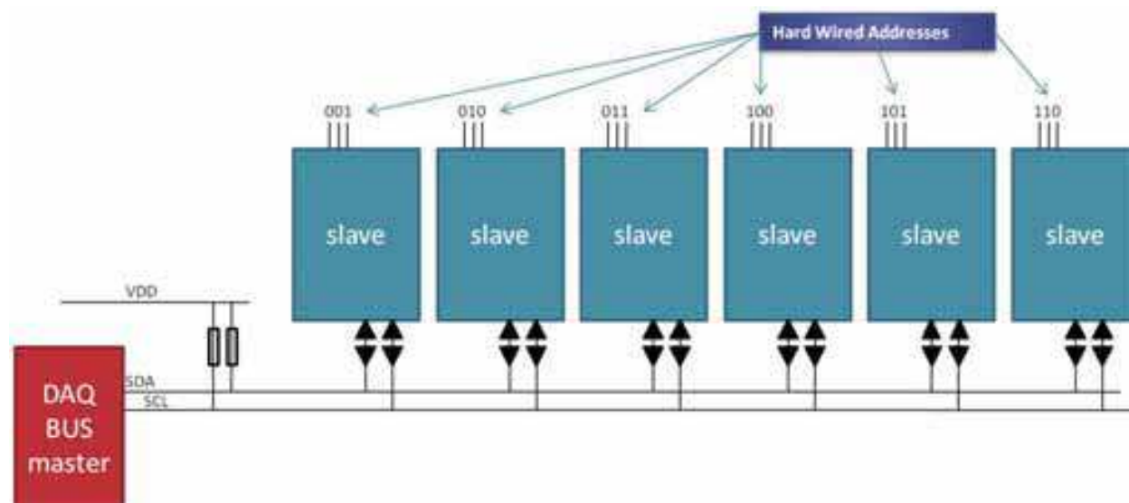
Fig. 23. I²C bus scheme.
