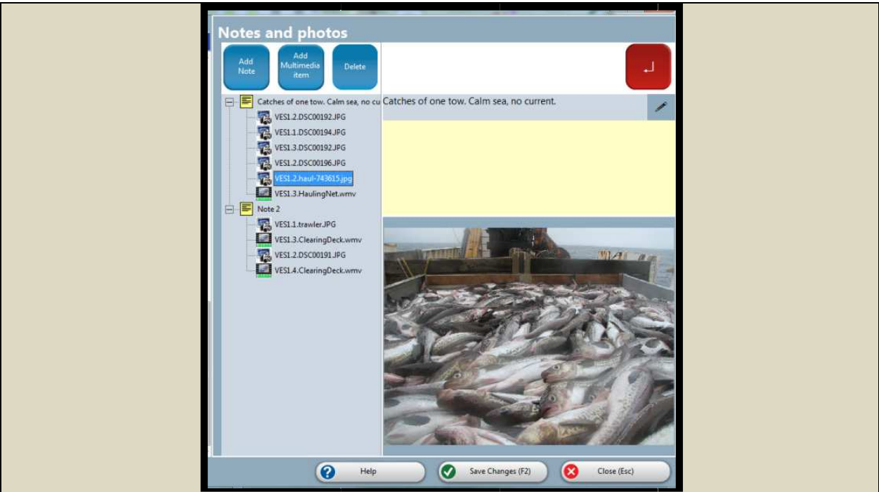
Fig. 15. Multinote Taker
