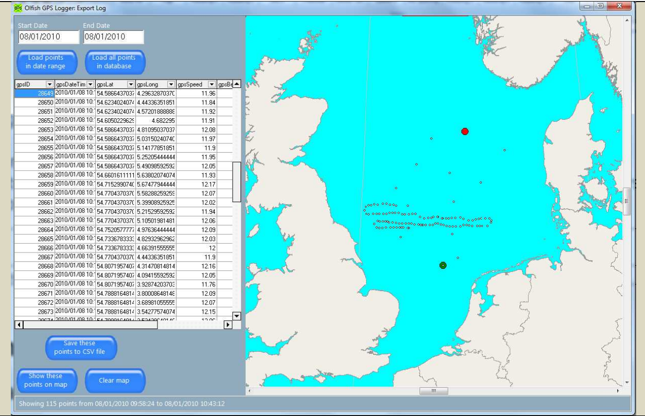
Fig. 7. GPS-Logger
