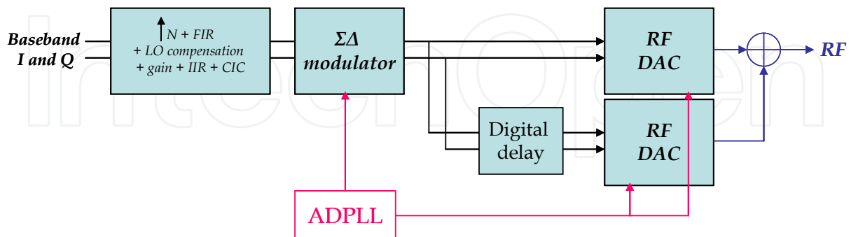
Fig. 22. Sigma Delta - RF-DAC architecture [Pozsgay et al]
