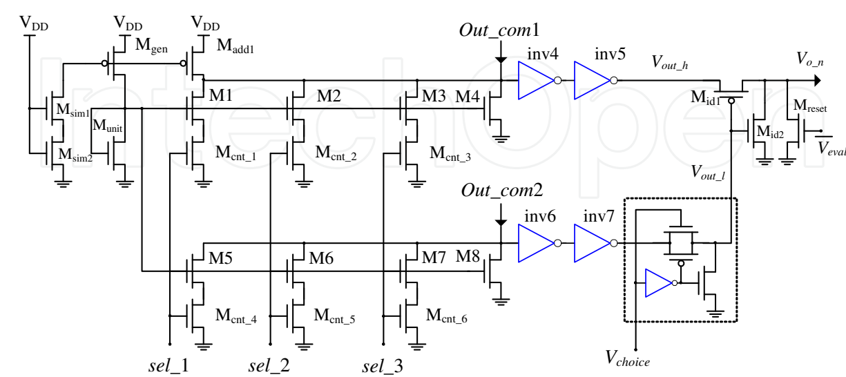
Fig. 20. Evaluation cell.
