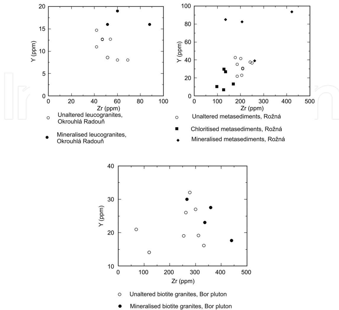
Figure 7. Plot Y versus Zr for unaltered and mineralised rocks from the Okrouhlá Radouň, Rožná and Zadní Chodov uranium deposits.
