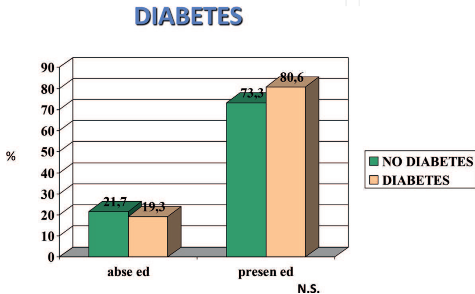
Graph 3. Diabetes%. N.S.
