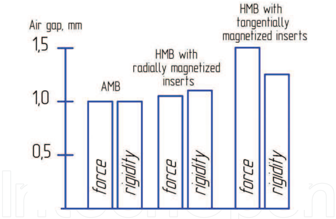
Figure 9. Comparison of the AMB parameters and various HMB designs.
