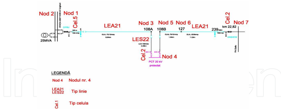
Figure 7. 20 kV OEL Ungheni-Cipău.
