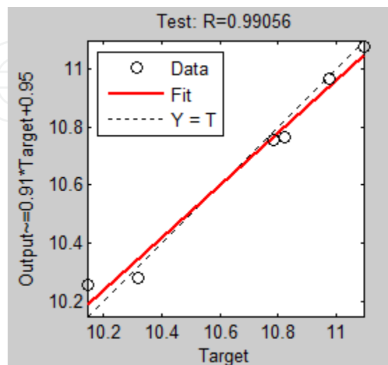
Figure 24. Jatropha OBM Validation values
