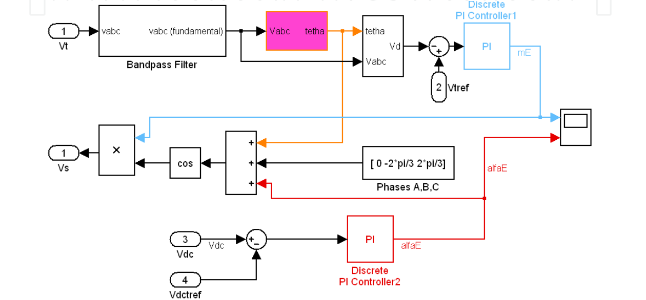
Fig. 18. Shunt controller.
