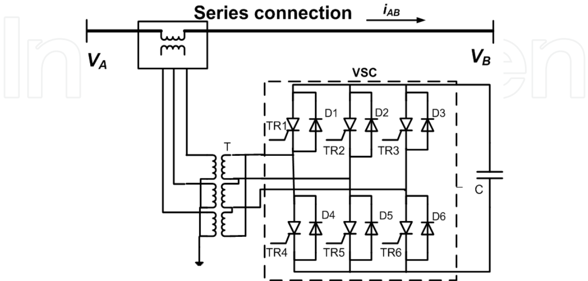
Fig. 7. SSSC
