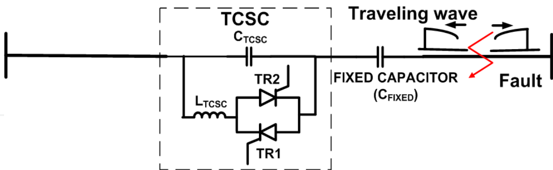
Fig. 14. TCSC controller
