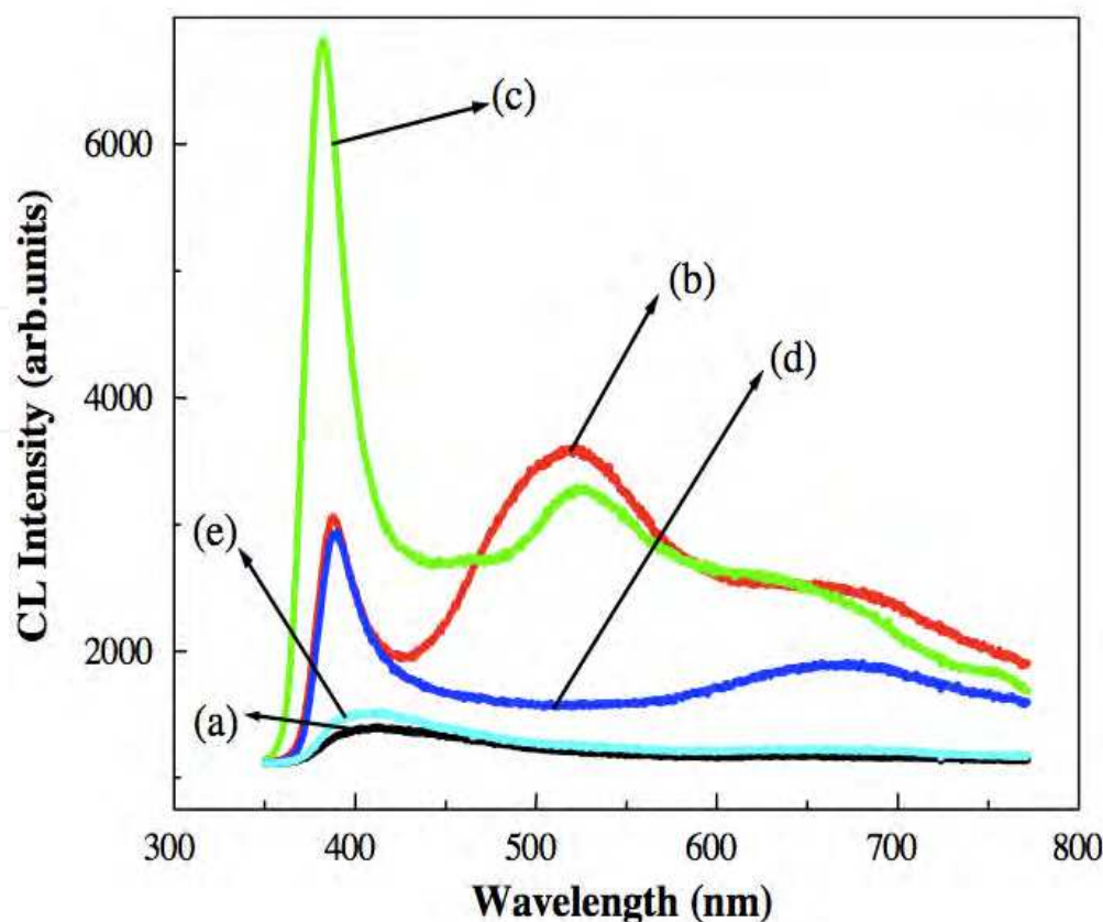
Fig. 5. CL Spectra of ZnO deposited at 450°C for different flow rate : (a) : f= 2,5\text{ml/ min} , (b) : f= 3.75\text{ml/ min} , (c) : f= 5\text{ml/ min} , (d) : f= 6.25\text{ml/ min} and (e) : f= 7.5\text{ml/ min}
