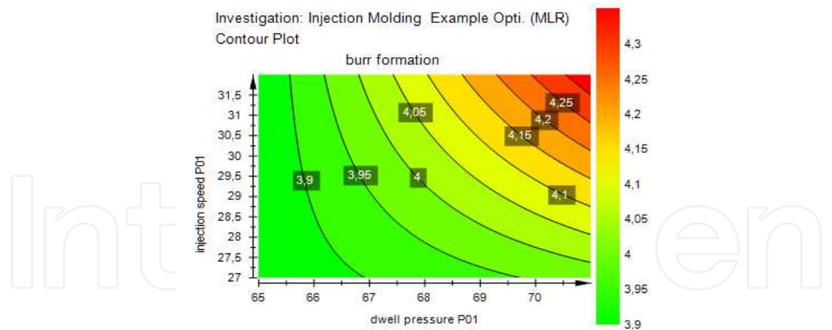
Fig. 29. Contour plot 5 .
