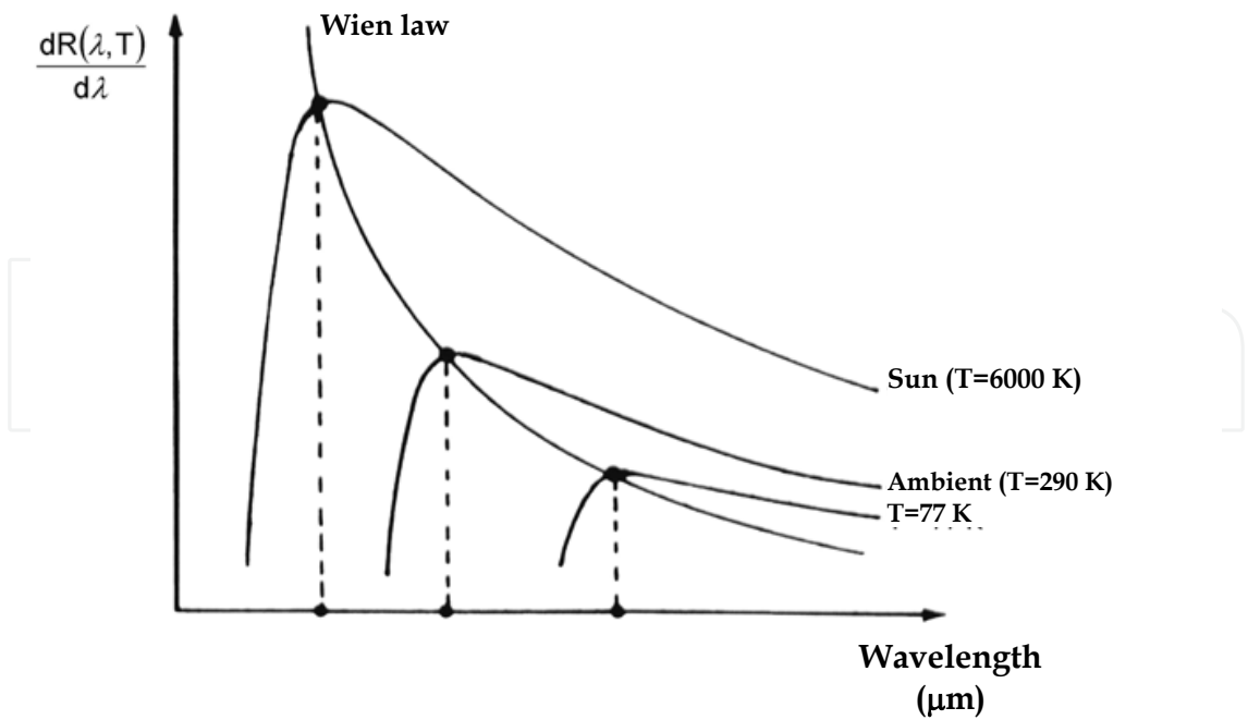
Fig. 4. Wien law (Gaussorgues, 1999).
