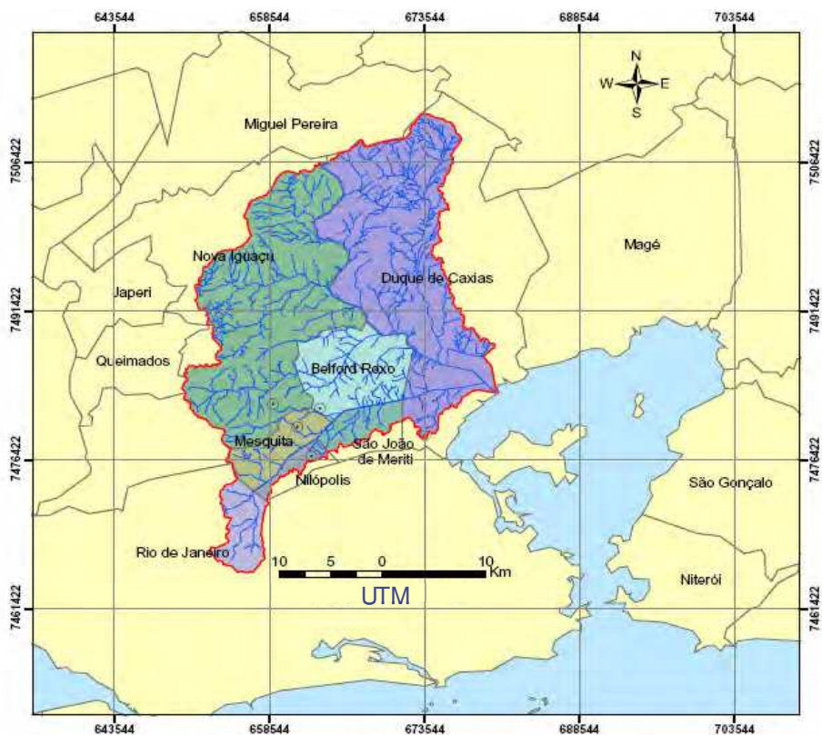
Fig. 6. Iguaçu-Sarapuí River Basin at Baixada Fluminense Lowlands in the Metropolitan Area of Rio de Janeiro.
