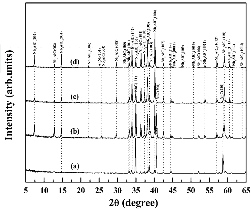
Fig. 12. Effect of initial element compositions (molar ratio of Nb, Al, and C) on the synthesis of Nb 4 AlC 3 : (a) 4 : 1.1 : 2.7, (b) 4 : 1.3 : 2.7, (c) 4 : 1.4 : 2.7, and (d) 4 : 1.5 : 2.7 [5].
