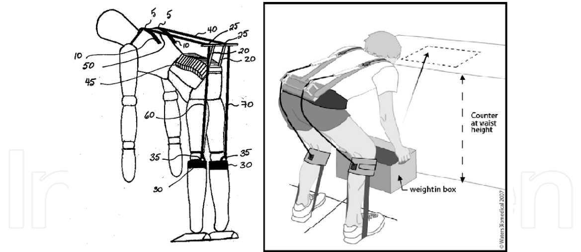
Fig. 10. PLAD lift assist system.
